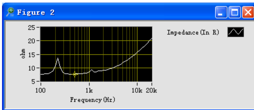
图 5 阻抗
