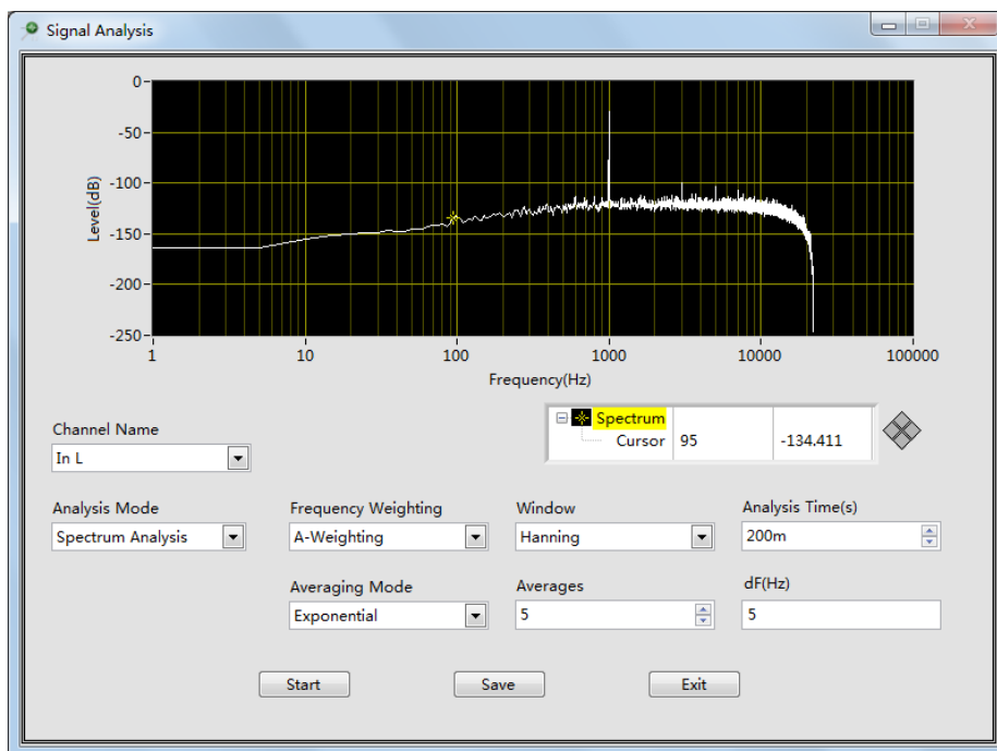
图 9 频谱分析
