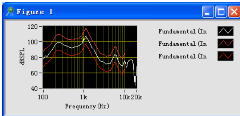
图 3 频率响应
