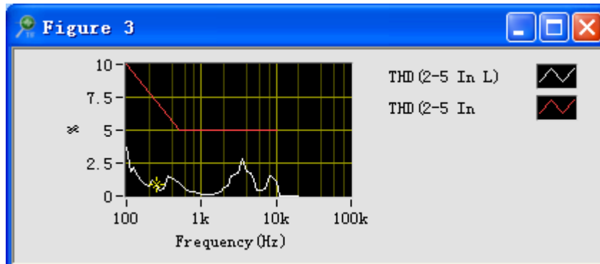
图 4 THD
